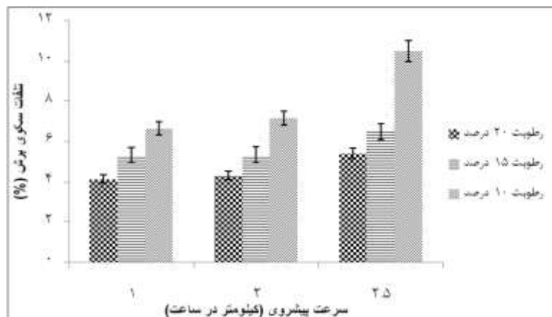
نمودار ۲ اثر متقابل سرعت پیشروی و رطوبت بذر بر تلفات سکو برش
