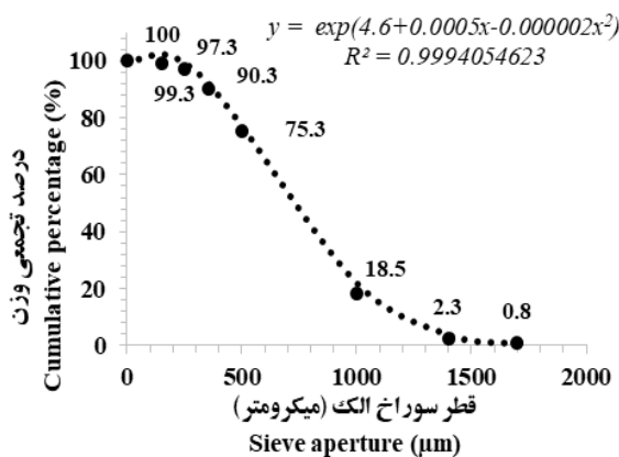
شکل (۴) نمودار درصد تجمعی میزان شکر باقی مانده
