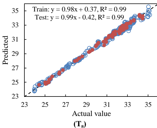
شکل ۸- مقایسه بین مقادیر واقعی و پیش‌بینی شده ۴ متغیر داخلی گلخانه توسط مدل RBF
