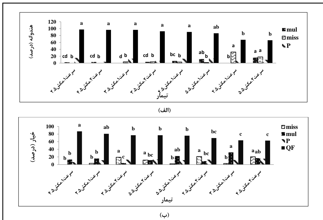
شکل ۶- مقایسه میانگین پارامترهای عملکردی بر شاخص‌های عملکردی مختلف برای الف) بذر خیار و ب) بذر هندوانه سرعت ۱: ۳ تا ۴ کیلومتر بر ساعت، سرعت ۲: ۶ تا ۸/۵ کیلومتر بر ساعت و مکش بر حسب کیلوپاسکال (شاخص چندگانه کاشت: mul، شاخص نکاشت: miss، شاخص کیفیت کاشت: Qf، شاخص دقت در فاصله کاشت: P)
